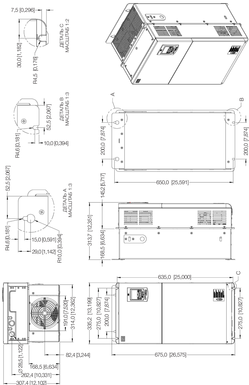
Рисунок В.11: Размеры преобразователя в мм [дюймах] - типоразмер G
