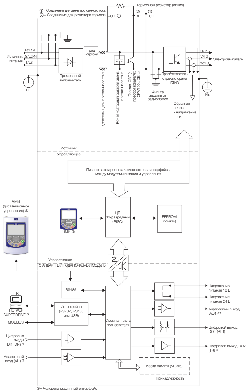
Рисунок 2.3: Блок-схема CFW500 - типоразмеры F и G
