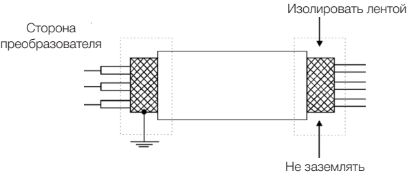
Рисунок 3.5: Подключение экрана кабеля
